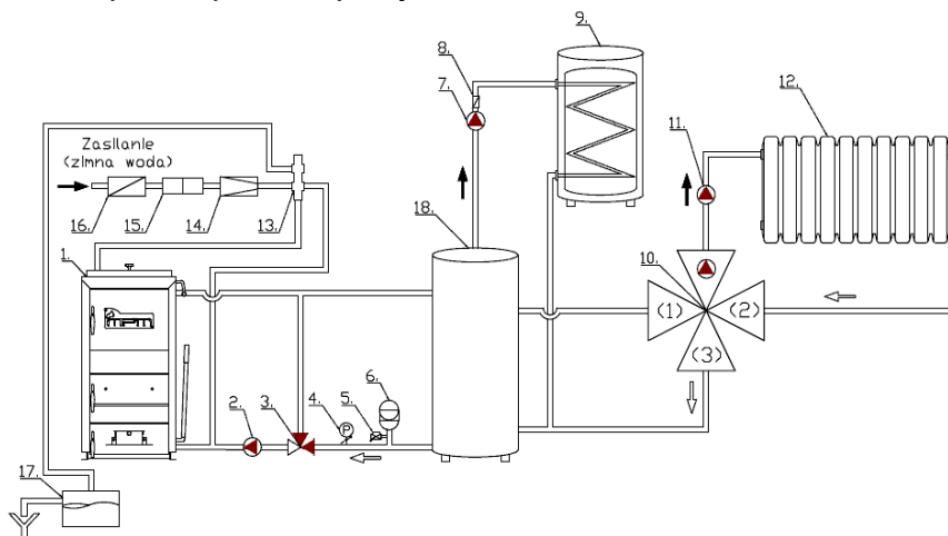
Rysunek 4. Przykładowy schemat podłączenia kotła MPM Wood Plus w układzie zamkniętym.
