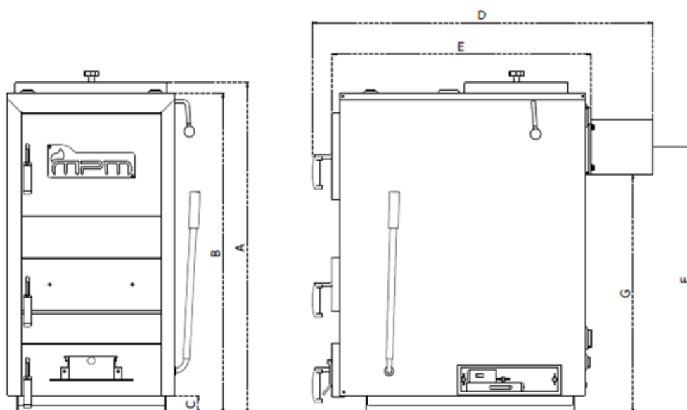
Rysunek 2. Podstawowe wymiary kotła MPM Wood Plus
